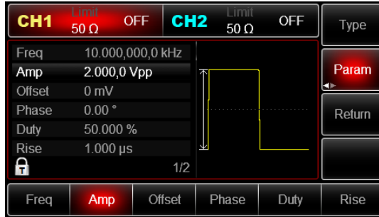
Figure 4- 26 Set rising edge
